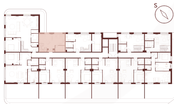
PÔDORYS PODLAŽIA
